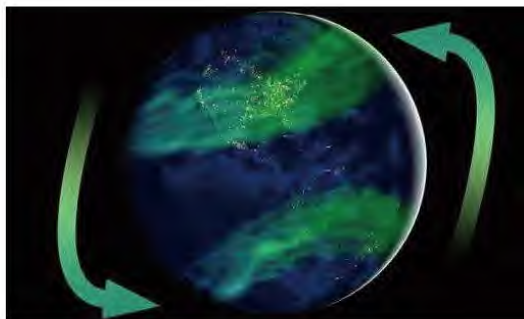
地磁场倒转（示意图） | 来自网络
