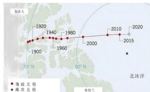
磁北极(这里应指北极磁极) 移动示意图 | 来自网络
